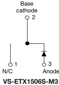
TO-263AB (D²PAK)
