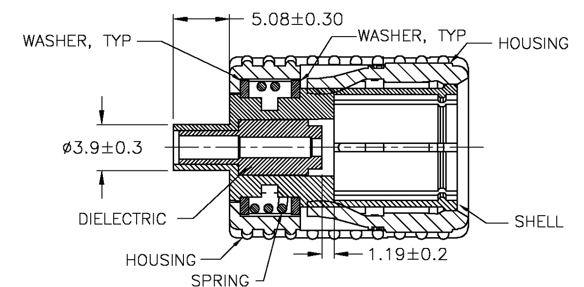
SECTION A-A 109763-3
