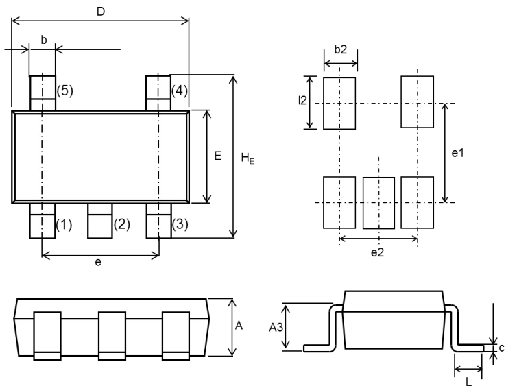
SOT-25T, (TSMD5)
