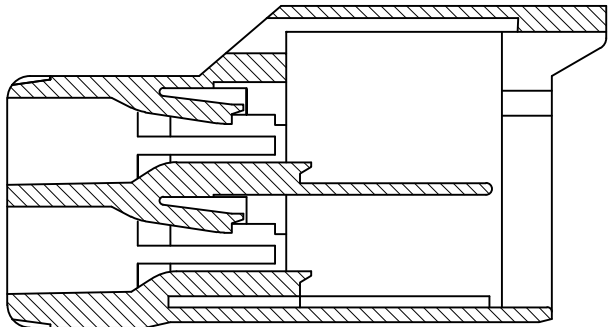
断面A-A
