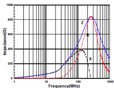
ACML-0402H-601
