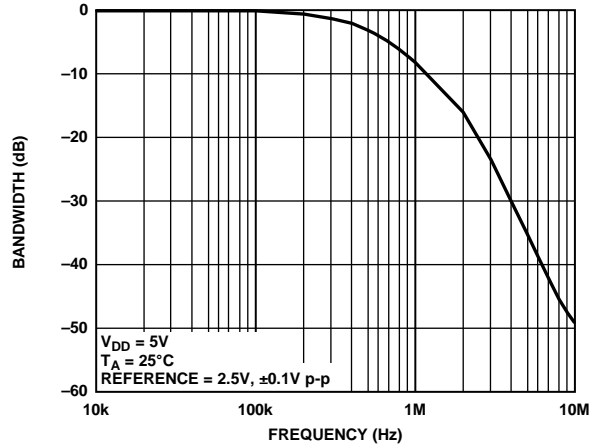
图40. 乘法带宽(外部基准电压源 = 2.5 V, \pm 0.1 V p-p, 10 kHz至10 MHz)
