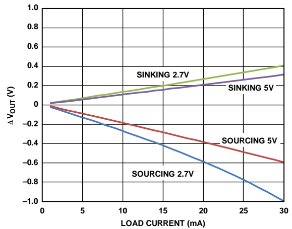
图31. 上裕量/下裕量与负载电流的关系
