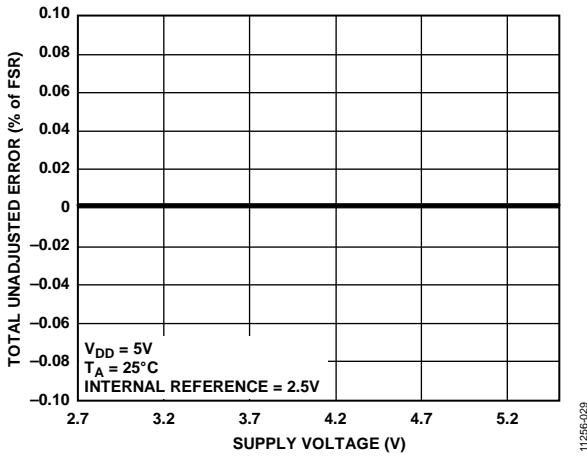
图27. TUE与电源的关系(增益=1)
