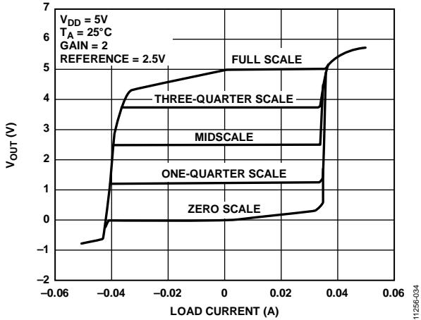
图32. 5 V时的源电流和吸电流能力(增益 = 2)
