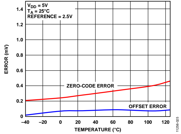
图23 零代码误差和偏置误差与温度的关系
