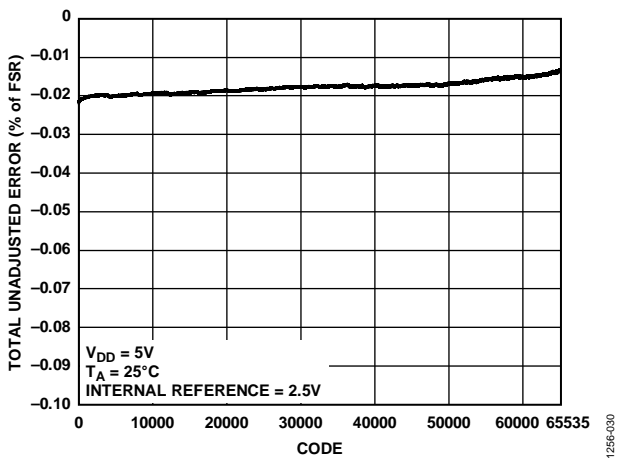
图28 TUE与代码的关系
