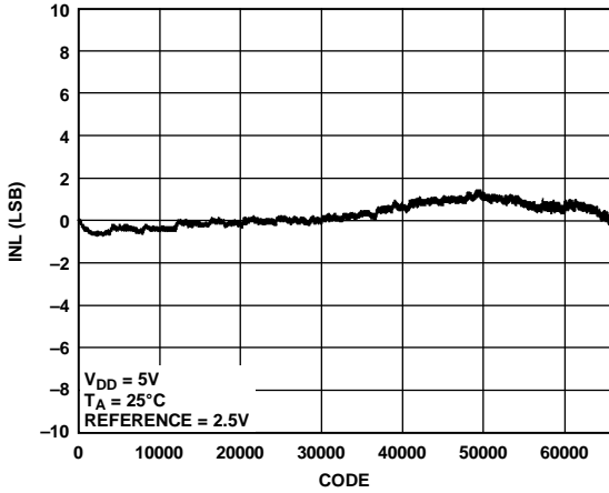
图14. AD5689R积分非线性(INL)与代码的关系
