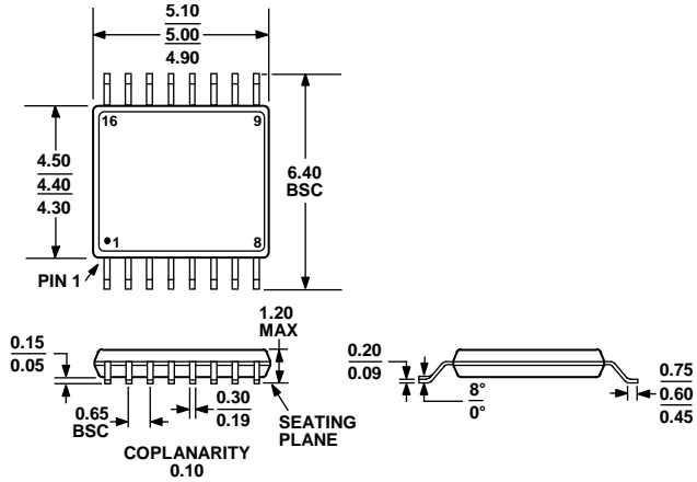
图55. 16引脚超薄紧缩小型封装[TSSOP] (RU-16) 图示尺寸单位: mm
