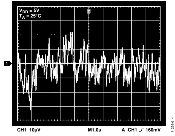
图12. 内部基准电压源噪声(0.1 Hz至10 Hz)
