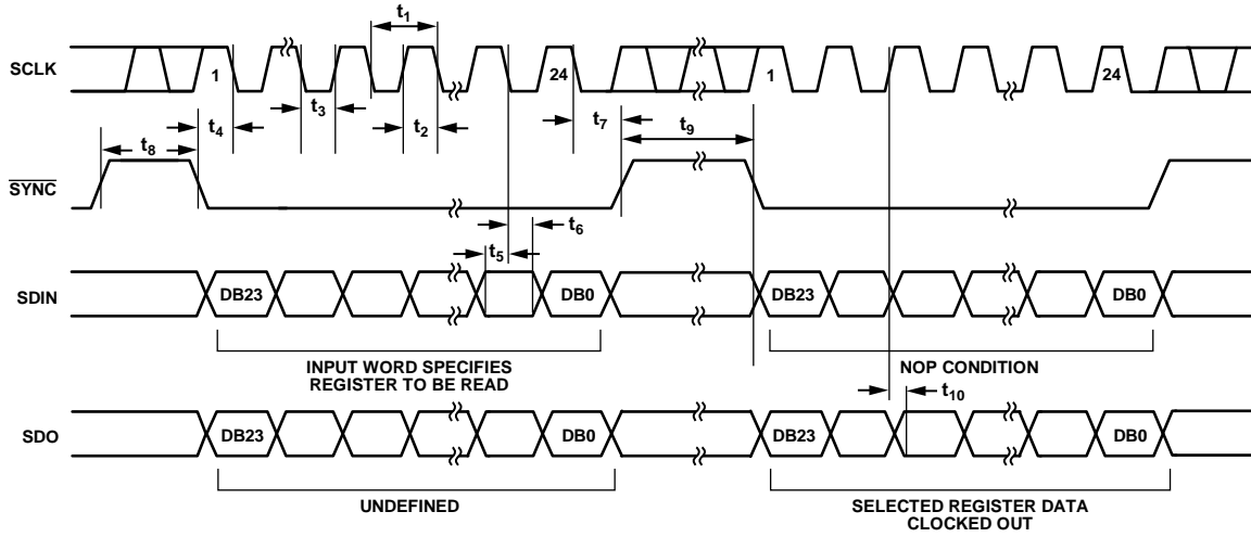
图5. 回读时序图
