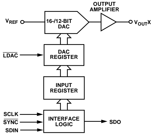
图47 单个DAC的输入加载电路示意图
