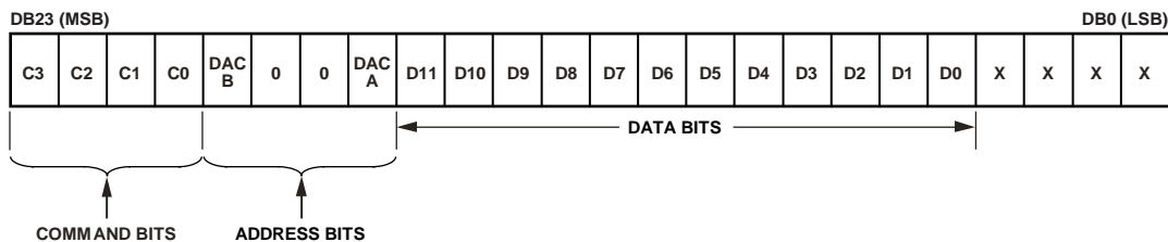
图44. AD5687R输入移位寄存器内容
