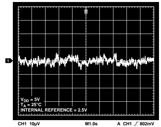
图37. 0.1 Hz至10 Hz输出噪声图, 2.5 V内部基准电压源
