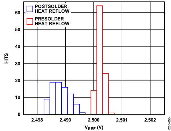
图48. SHR基准电压偏移
