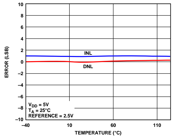
图19. INL误差和DNL误差与温度的关系
