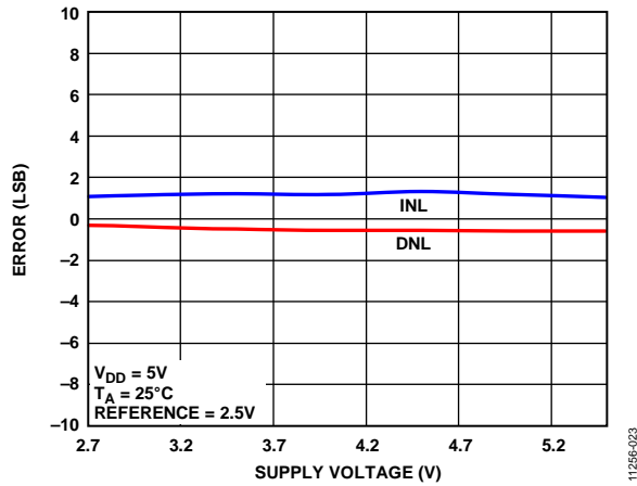
图21. INL误差和DNL误差与电源电压的关系
