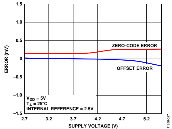
图25. 零编码误差和偏置误差与电源电压的关系
