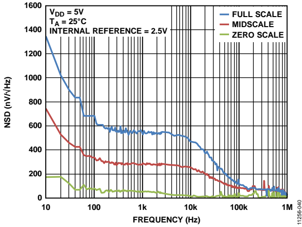
图38. 噪声频谱密度(NSD)
