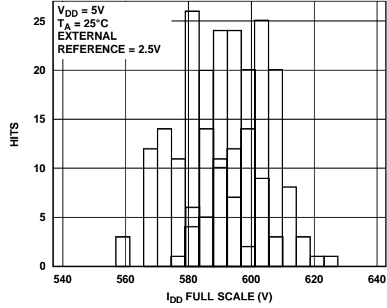
图29. 采用外部基准电压源时的 I_{DD} 直方图( V_{DD} = 5V )
