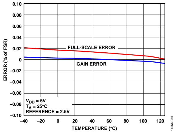
图22. 增益误差和满量程误差与温度的关系
