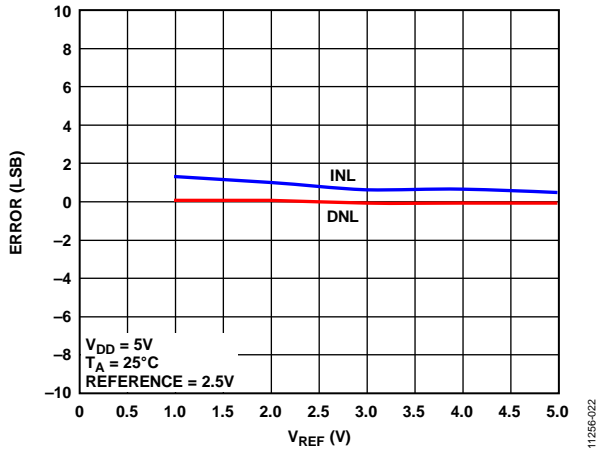
图20. INL误差和DNL误差与 V_{REF} 的关系
