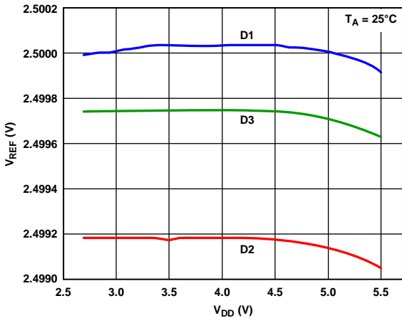
图16. 内部基准电压与电源电压的关系
