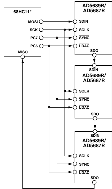
图45. 以菊花链方式连接多个AD5689R/AD5687R器件
