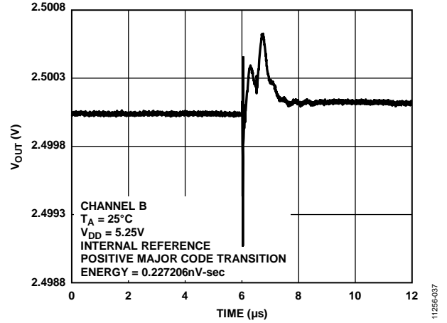
图35. 数模转换毛刺脉冲
