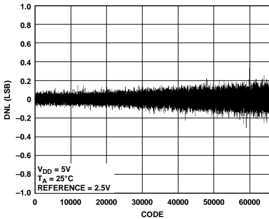
图15. AD5689R差分非线性(DNL)与代码的关系
