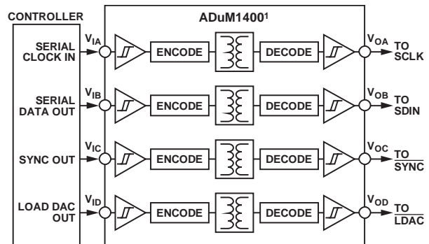
图53. 隔离接口
