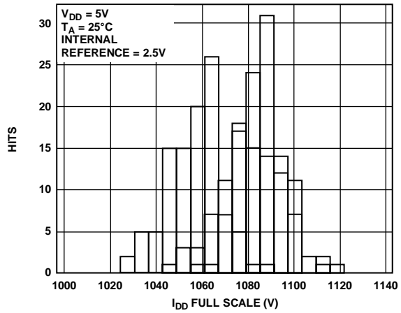
图30. 采用内部基准电压源时的 I_{DD} 直方图( V_{REF} = 2.5V , 增益=2)
