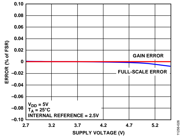
图24 增益误差和满量程误差与电源的关系
