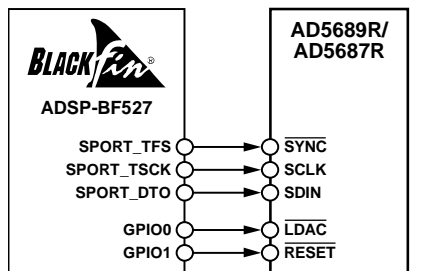
图51. AD5689R/AD5687R与SPORT接
