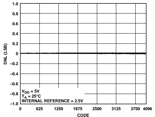
图18. AD5687R DNL与代码的关系
