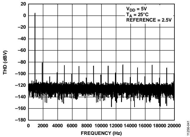
图39. 1 kHz时的总谐波失真
