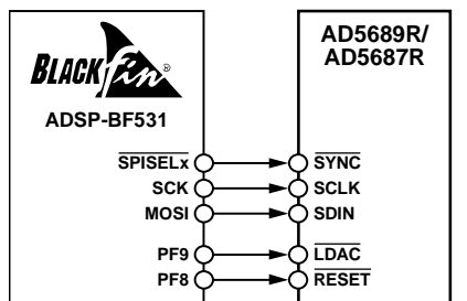
图50. ADSP-BF531与AD5689R/AD5687R接口
