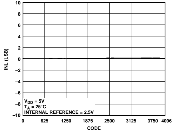
图17. AD5687R INL与代码的关系
