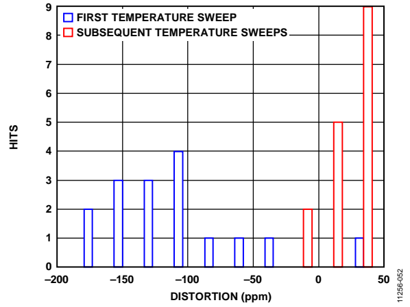
图49. 热滞
