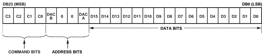
图43. AD5689R输入移位寄存器内容
