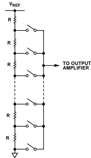
图42. 电阻串结构
