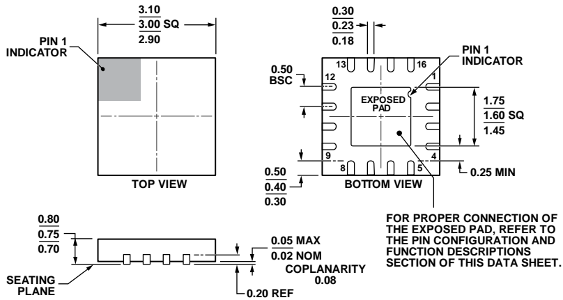
图54. 16引脚引线框芯片级封装[LFCSP_WQ] 3 mm x 3 mm超薄体 (CP-16-22) 图示尺寸单位: mm
