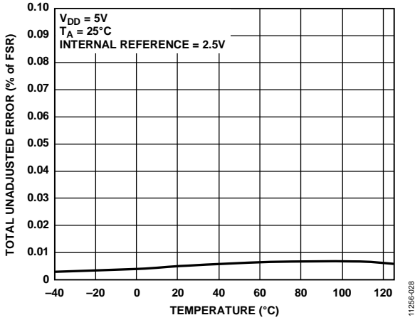
图26. 总不可调整误差(TUE)与温度的关系
