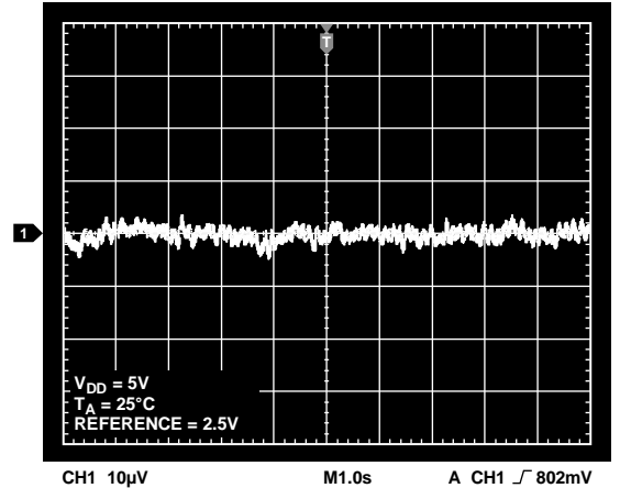
图36. 0.1 Hz至10 Hz输出噪声图, 外部基准电压源
