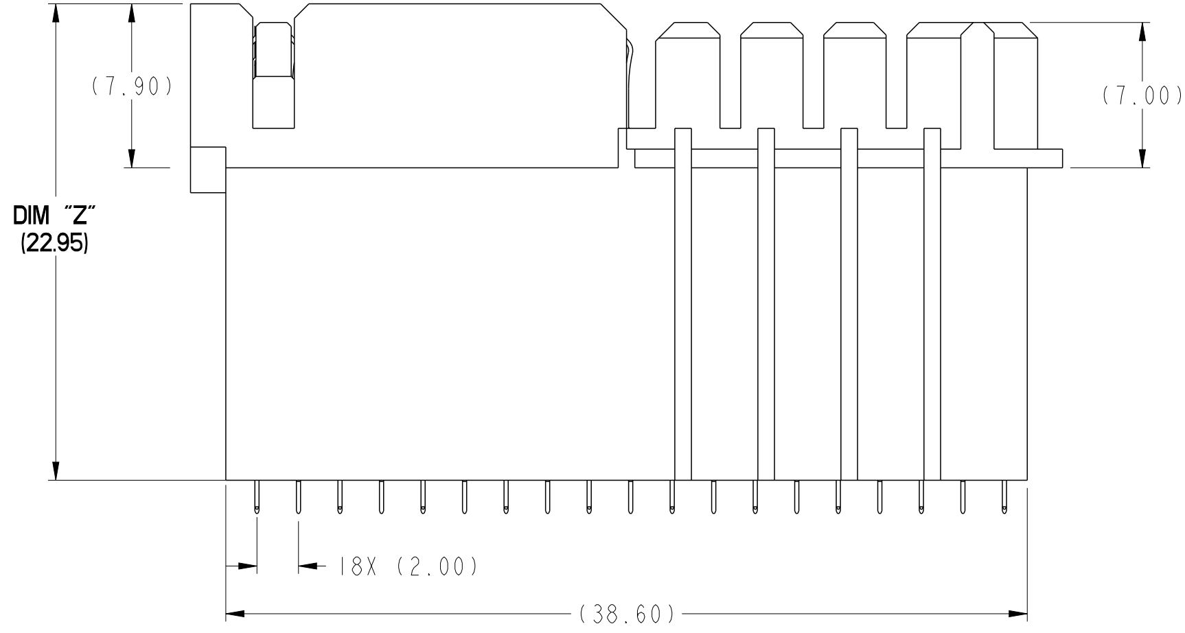
10127225-119500ULF SHOWN SCALE 4:1
