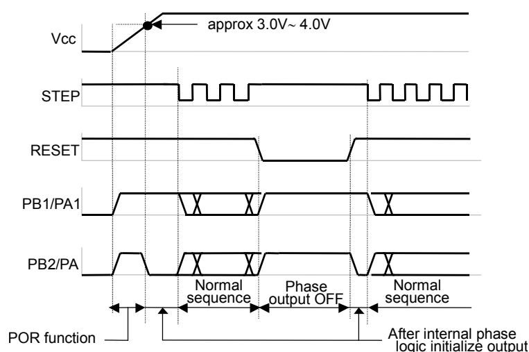
Fig.5 POR and external reset timing
