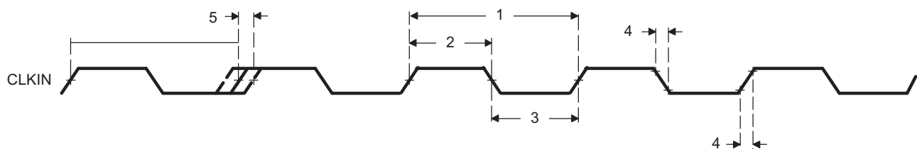
Figure 6-8. CLKIN2 Timing
