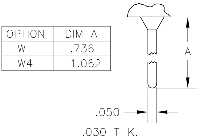
W W4 WIRE WRAP
