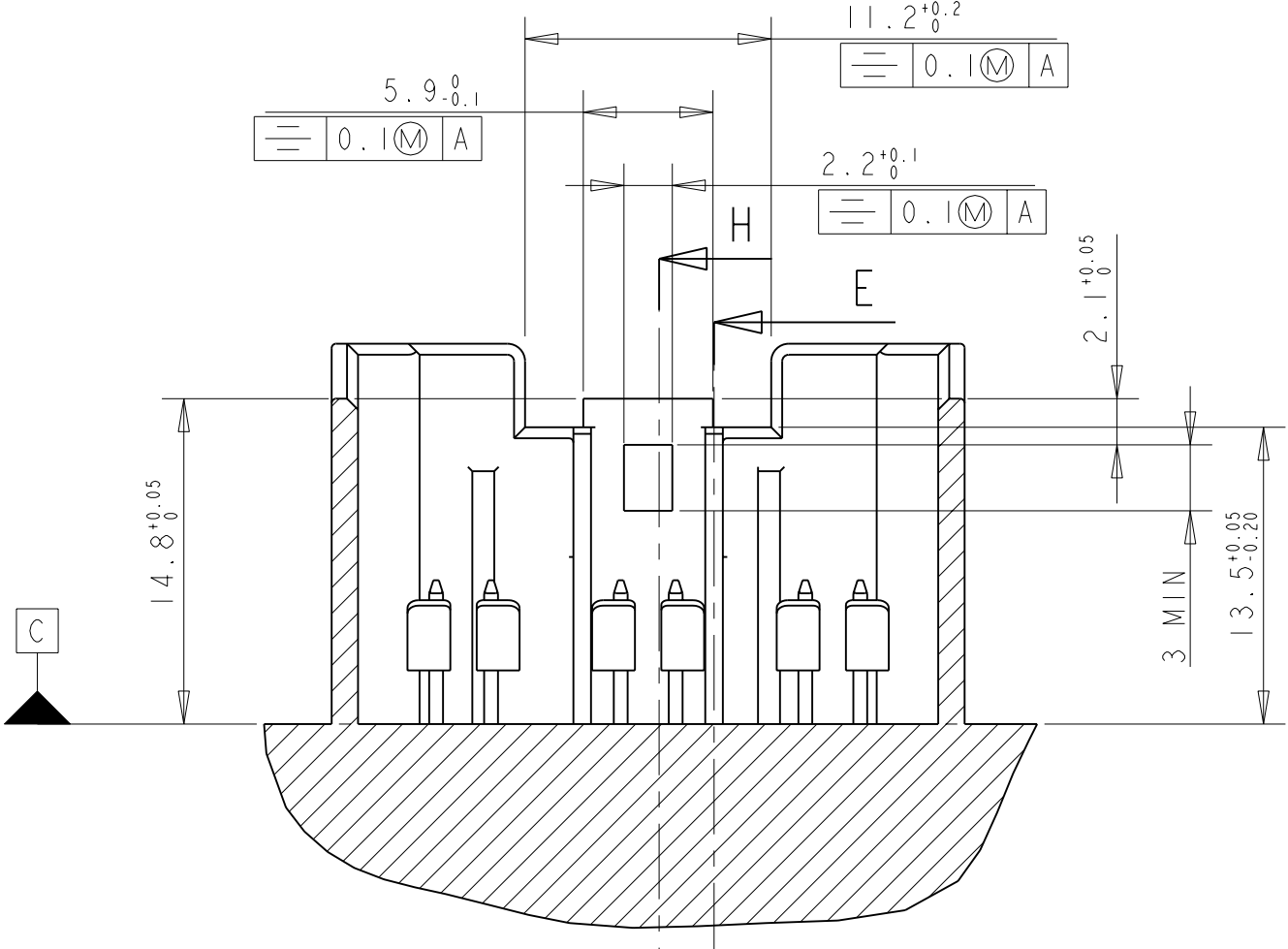
COUPE D-D
