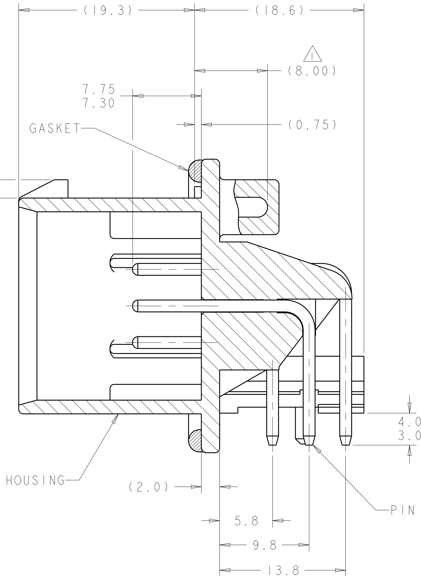
SECTION A-A
