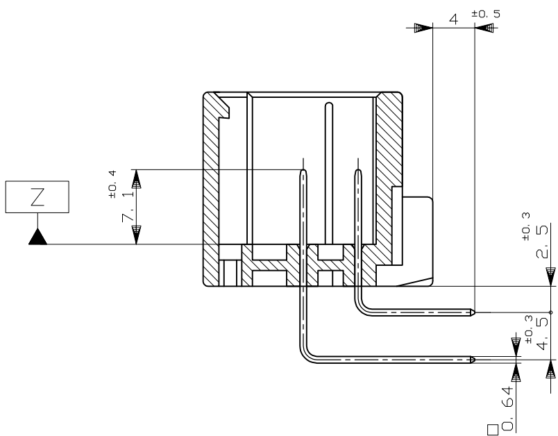
B-B
