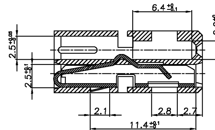
SECT A-A
