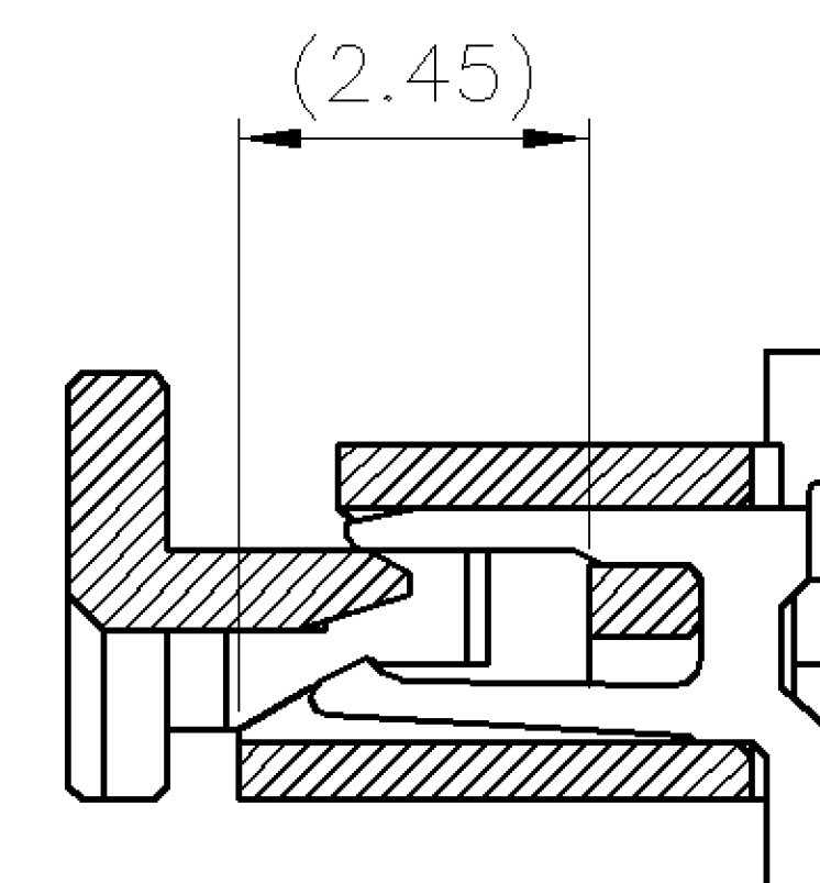
SECTION A-A
