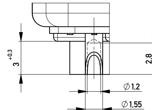
DETAIL X MAßSTAB 5 : 1
