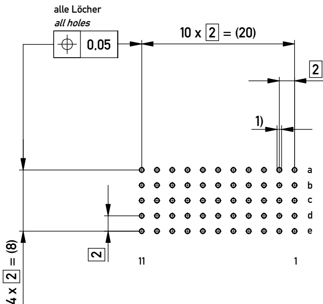
Lochbild für Leiterplatte (Bestückungsseite)
