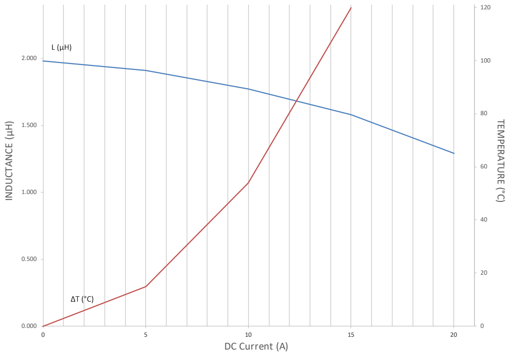
I&T Curve
