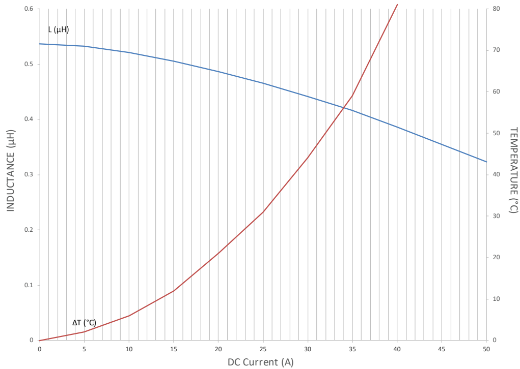
I&T Curve
