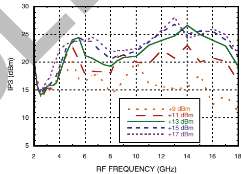
Input IP3 vs. LO Power, IF = 100 MHz
