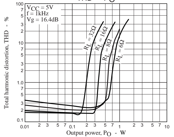
THD - P_O
