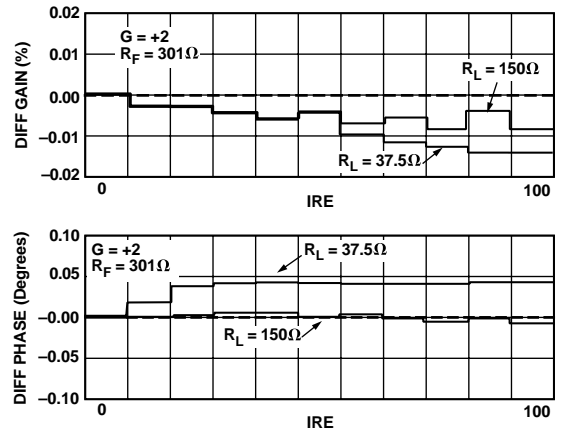
TPC 11. 差分增益和相位
