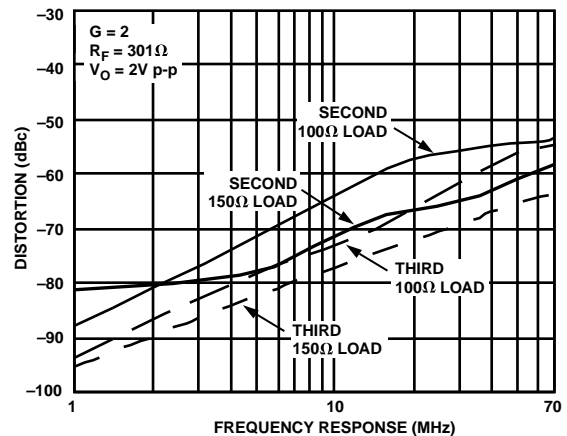
图2. 失真与频率的关系; G = +2
