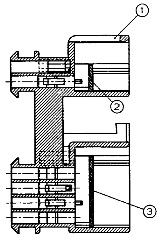
断面 A-A SECT.
