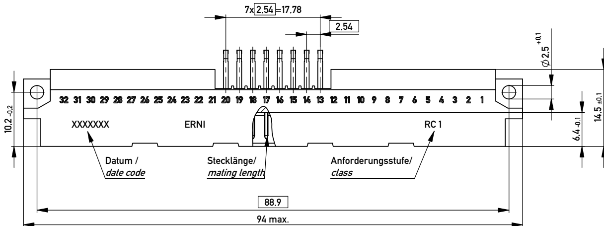
Bestückungsplan / contact layout
