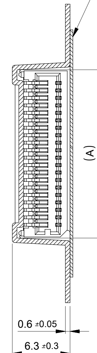
SECTION : Z-Z
