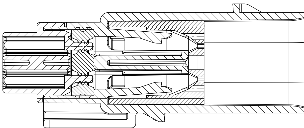
SECTION V-V
