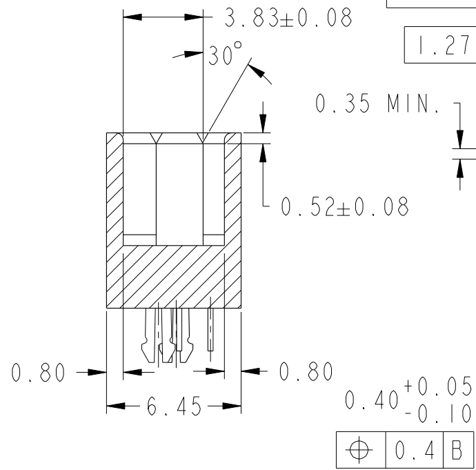
SECTION D-D
