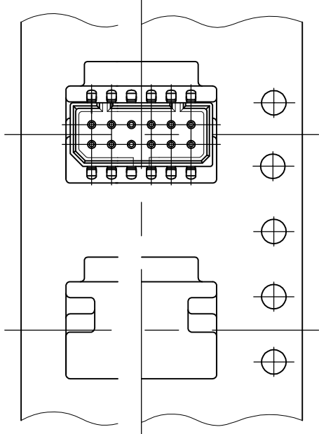
12 Pos. (P/N: 7-176890-2)
