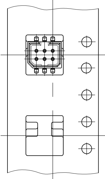
6 Pos. (P/N: 3-176890-6)
