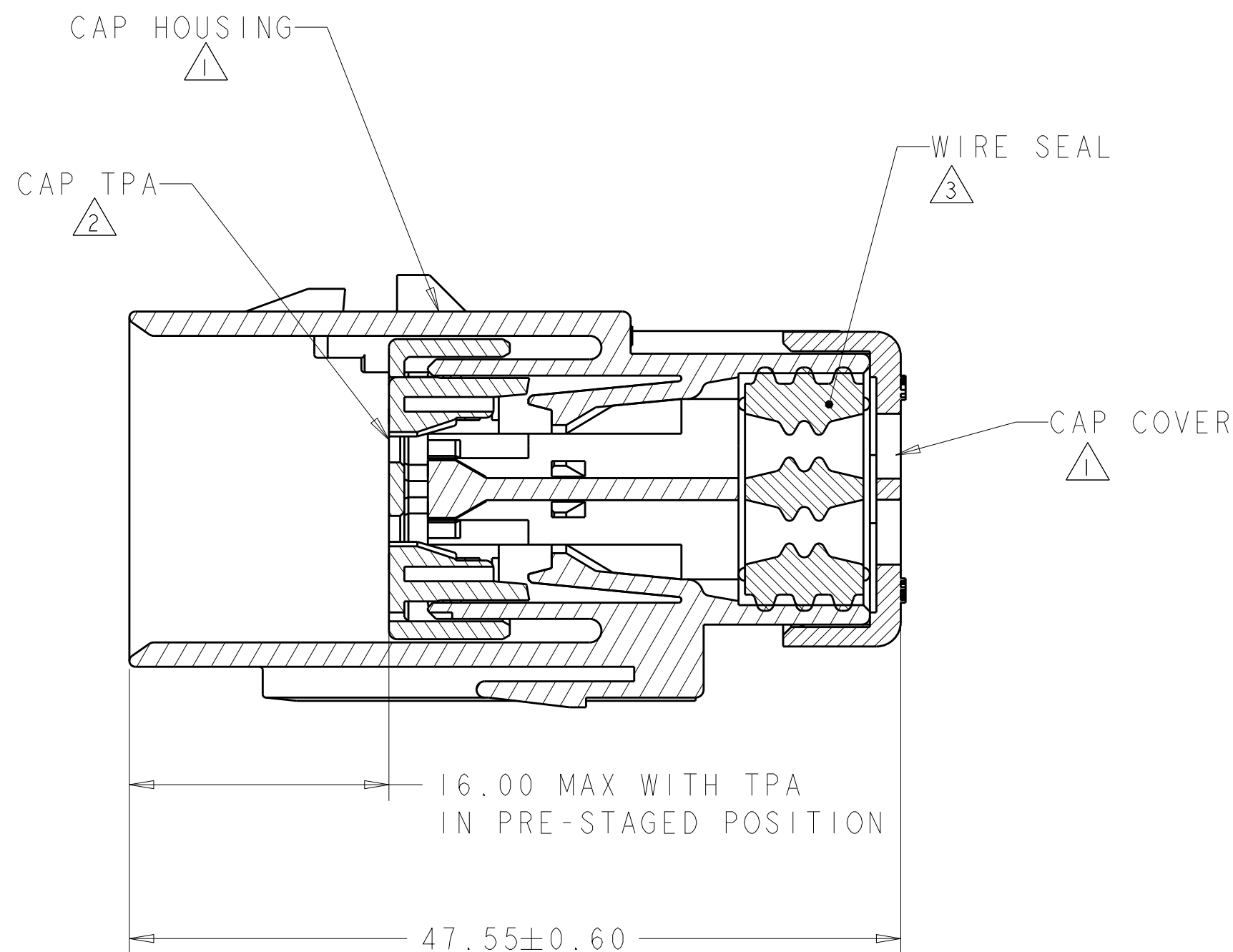
SECTION A-A
