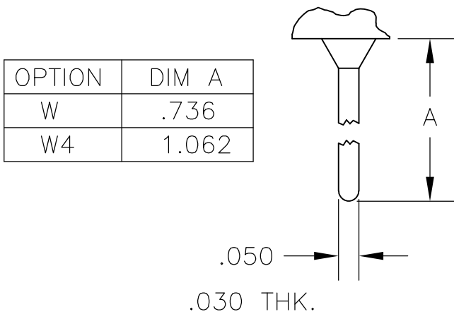
W W4 WIRE WRAP
