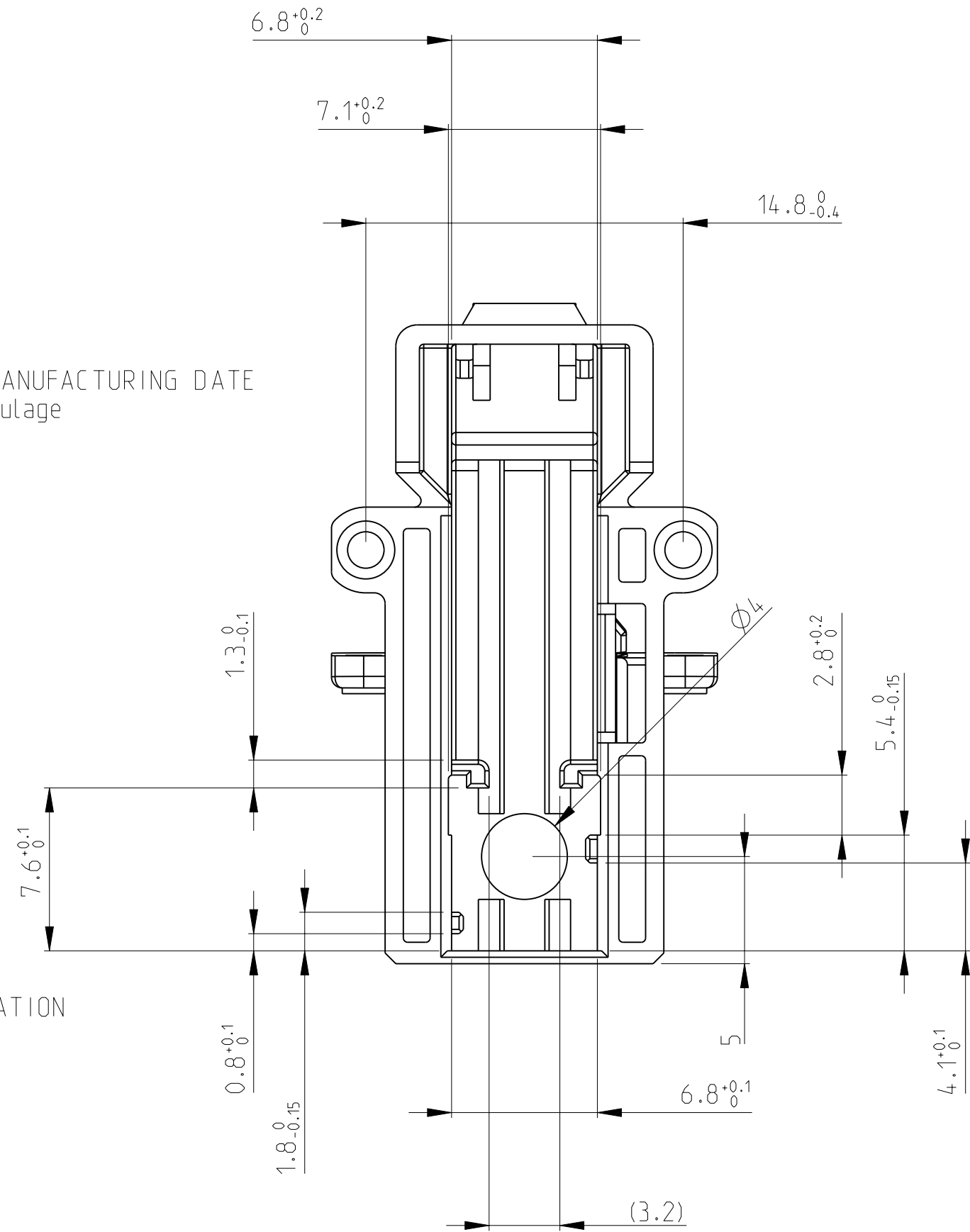
COUPE A-A
