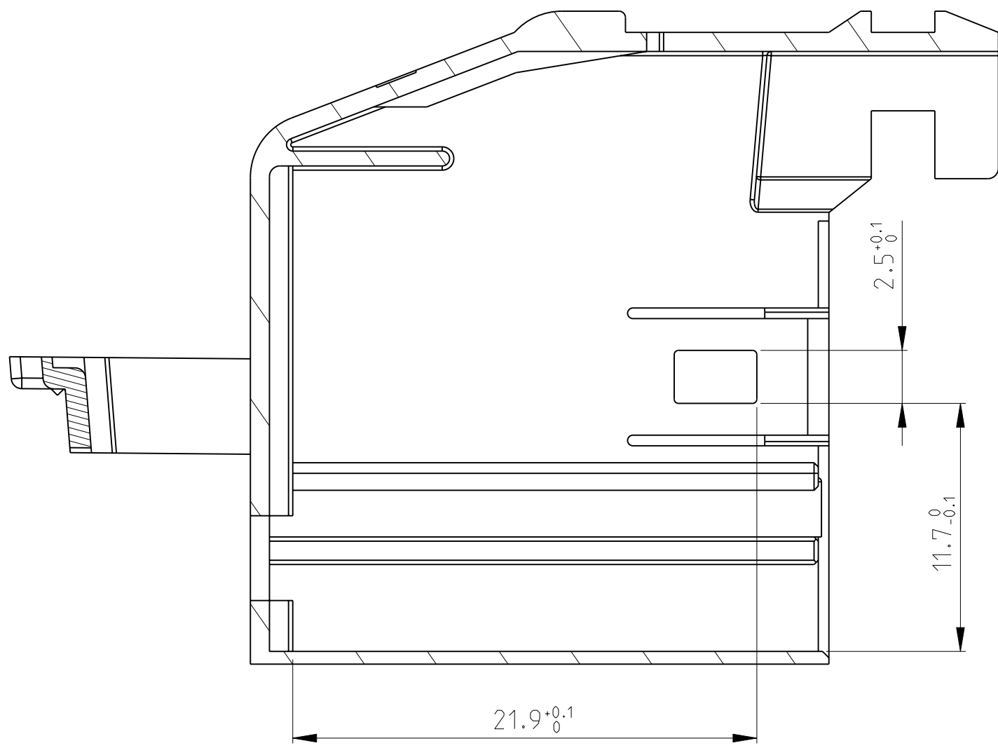
COUPE A-A
