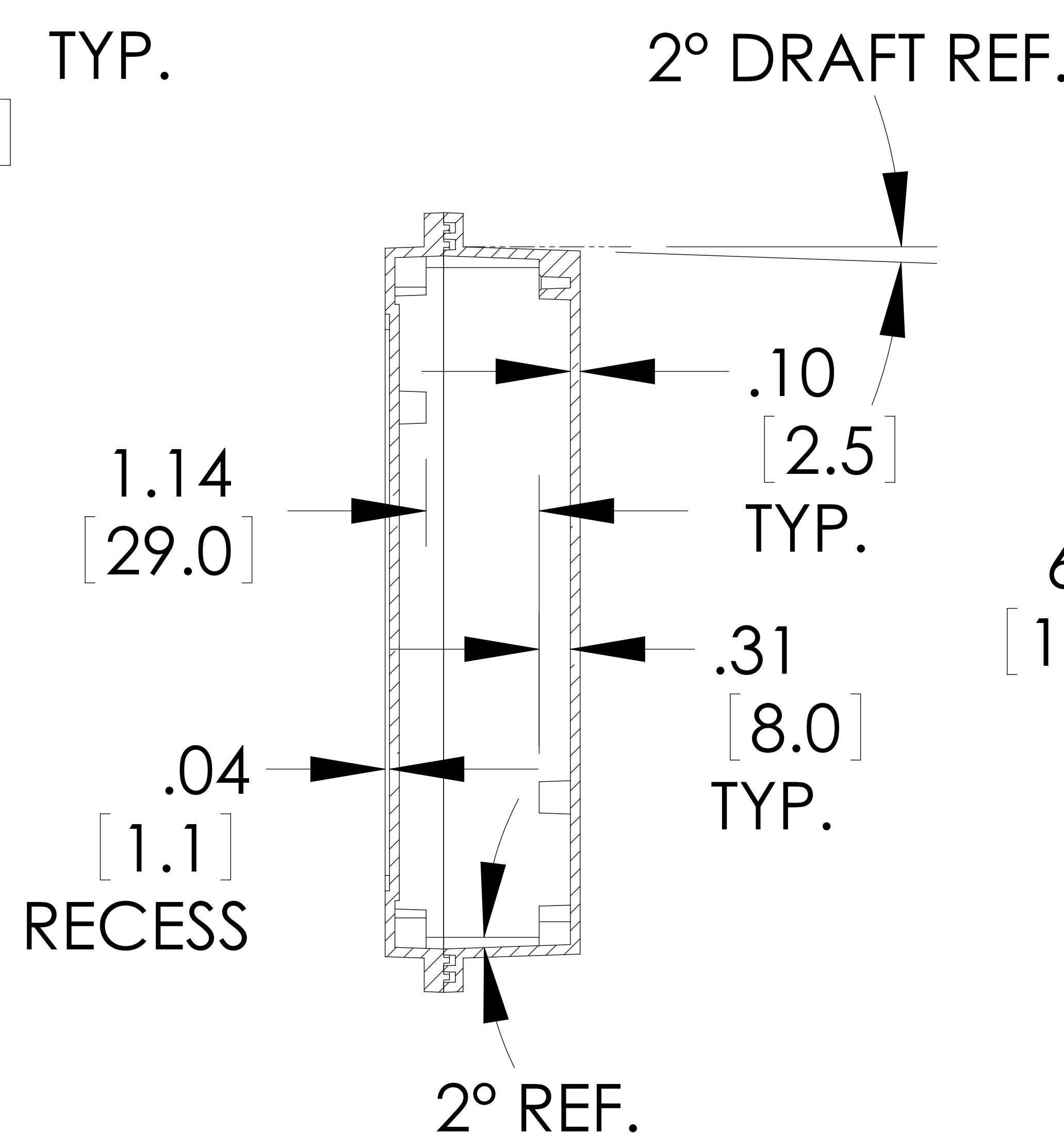
SECTION A-A
