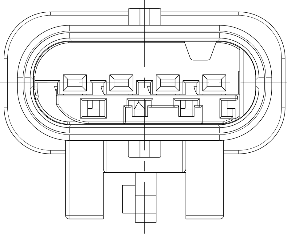
RETAINER MOVING DIRECTION 2.Kontaktsicherung Verschiebeweg
