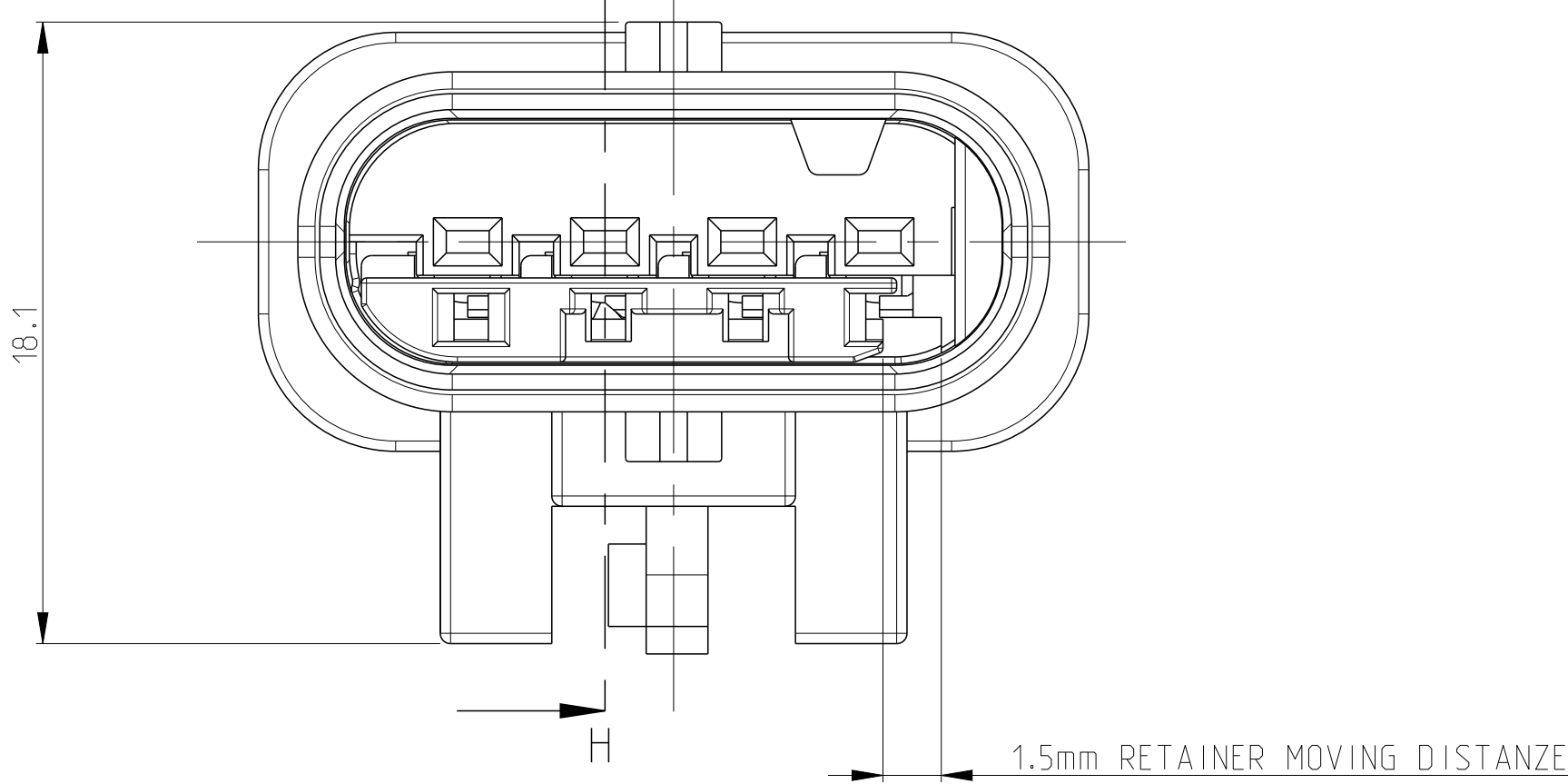
RETAINER IN PRE LOCKED POSITION Kontaktsicherung in Vorraststellung
