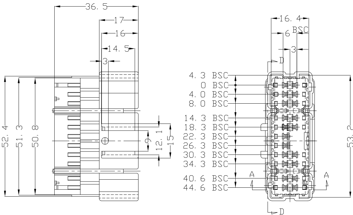
SECTION D-D
