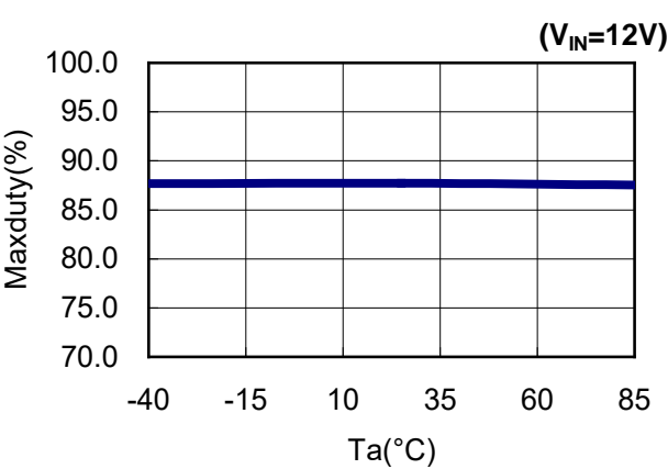
12) Maxduty(ver.A,B Rt=floating)
