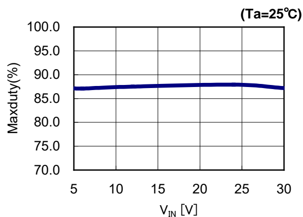
17) Maxduty(ver.G,H)
