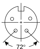
4 Pin 164-6040
