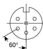
6 Pin 164-6060
