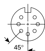
7 Pin 164-6070
