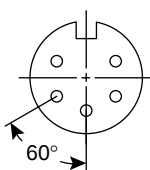
5 Pin 164-6051
