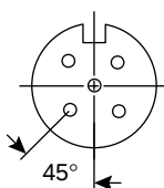
5 Pin Dice 164-6052
