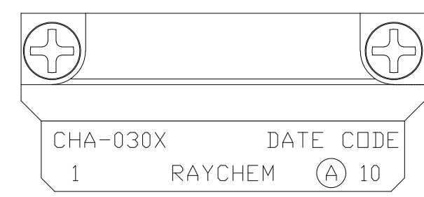
RECEPTACLE
