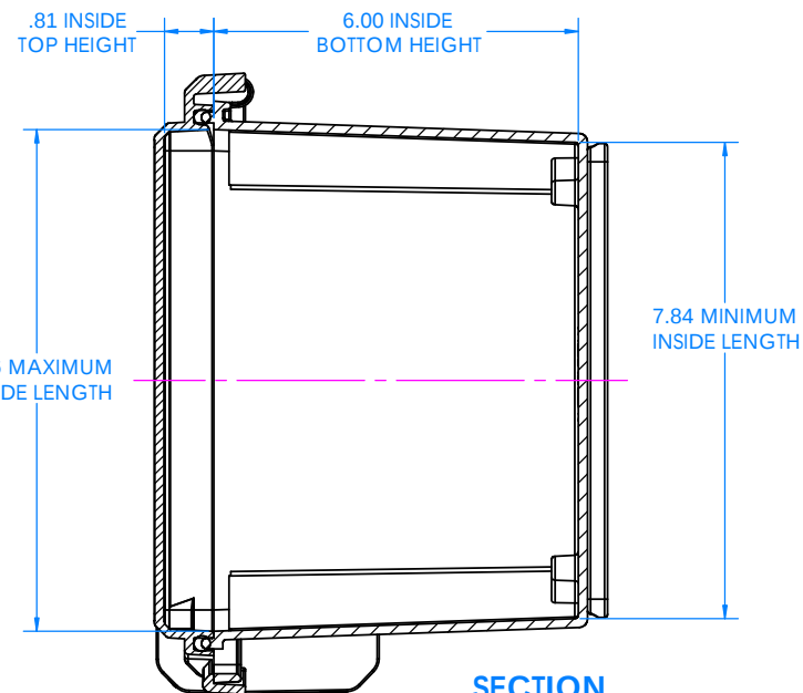
SECTION A-A SCALE 1 : 1.75
