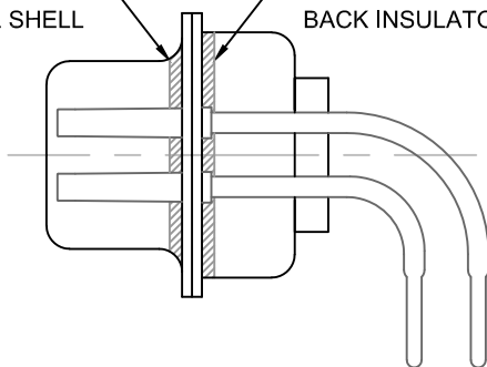
DETAIL A-A
