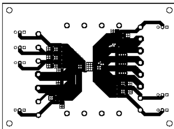
TOP Layer
