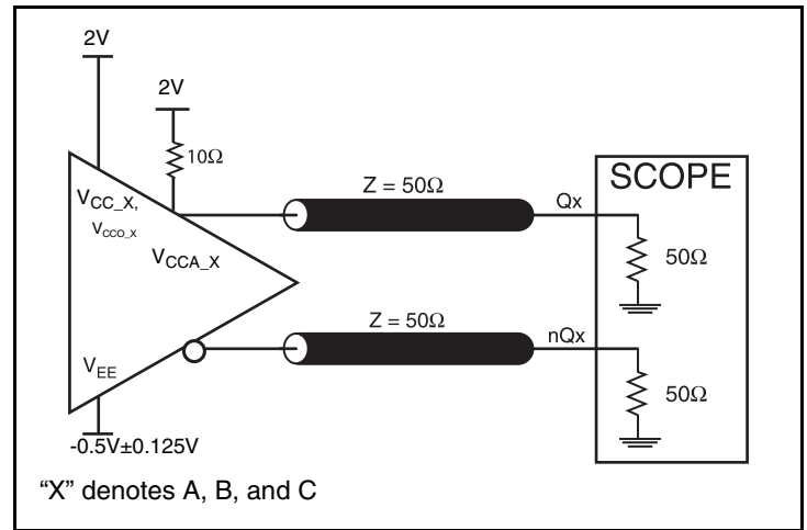
2.5V Core/2.5V LVPECL Output Load Test Circuit
