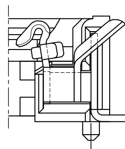
DETAIL E (SCALE 5:1)
