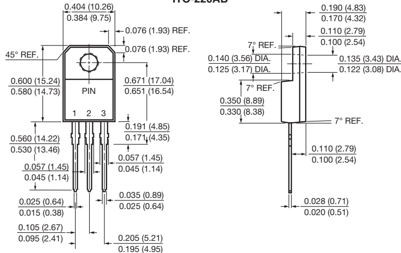
ITO-220AB
