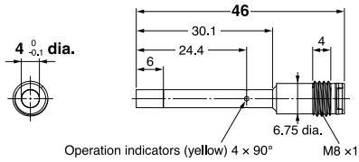
E2E-S05N03-MC-□□
