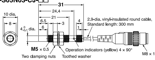
E2E-S05N03-CJ-□□
