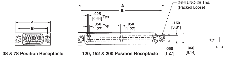
38 & 78 Position Receptacle
