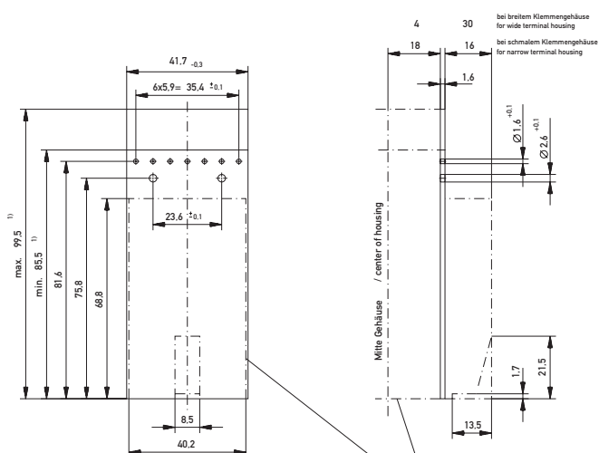
Längsplatine / Lengthwise circuit board
