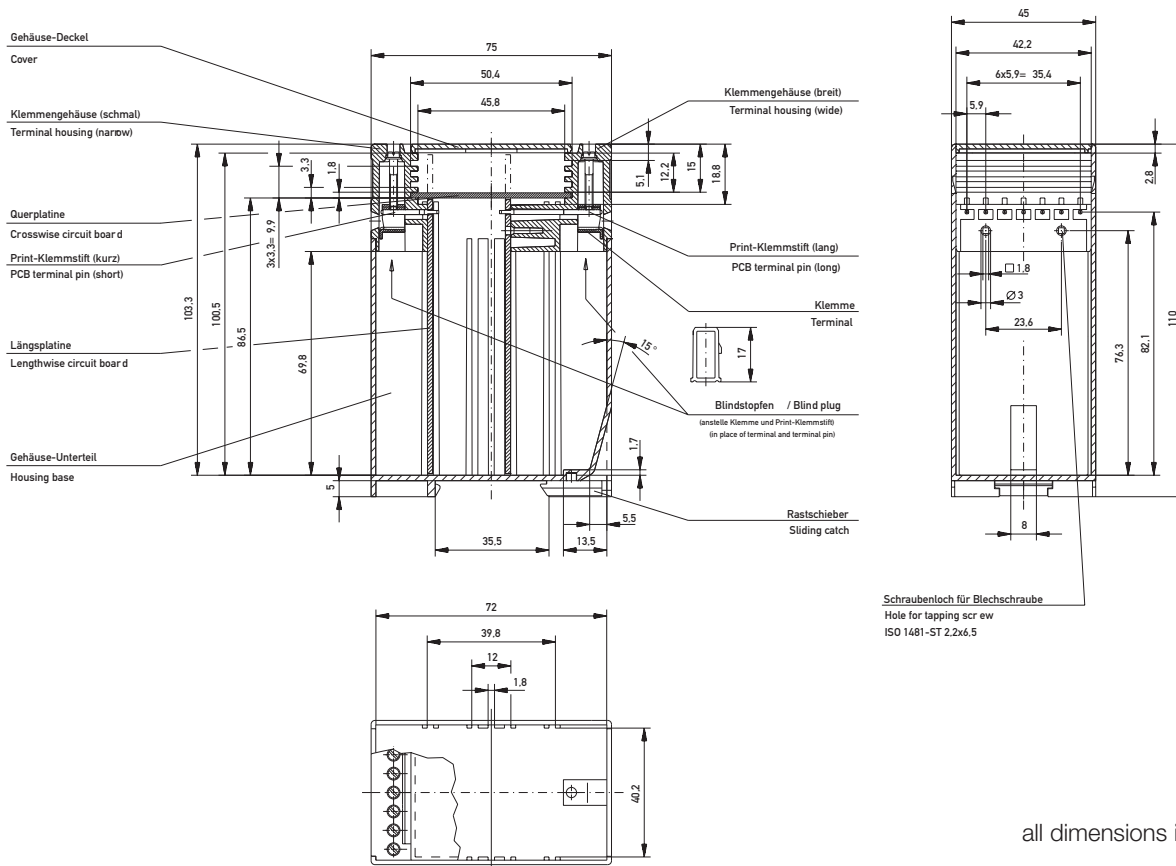
Längsplatine / Lengthwise circuit board
