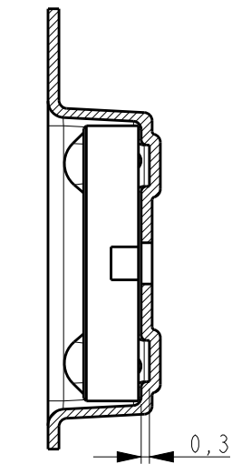
SECTION D-D
