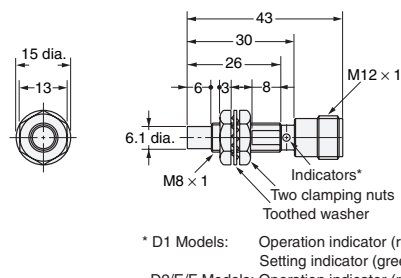
Diagram 19 E2E-X4MD□-M1(G) E2E-X2ME□-M1/E2E-X2MF□-M1
