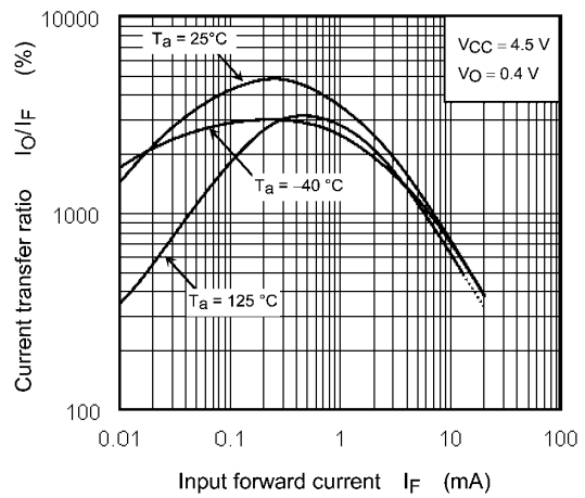
Fig. 12.2.8 I_O/I_F - I_F
