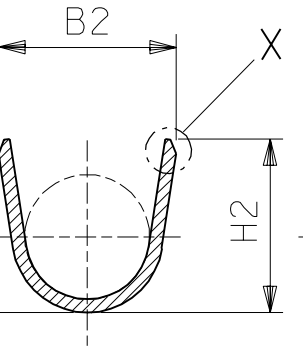
SECTION Z-Z SCHNITT Z-Z
