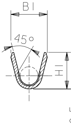
SECTION Y-Y SCHNITT Y-Y
