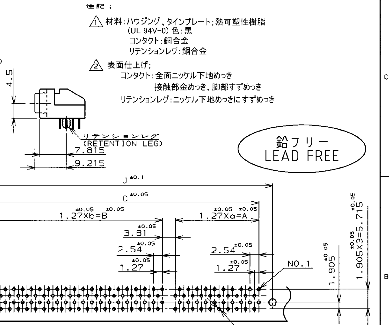
基板仕様 P.C. BOARD LAYOUT (コネクタ装着側) (CONNECTOR MOUNT SIDE)
